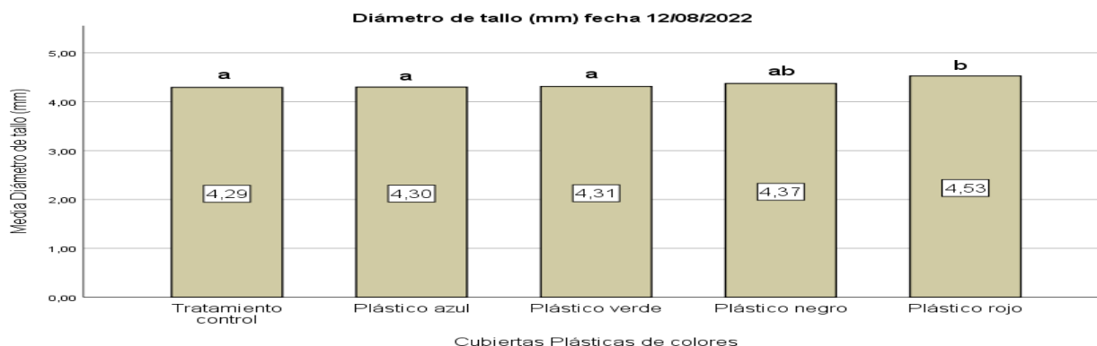
Figura 5. Promedio de diámetro de tallo a 25 ddt (12/08/2022), expresado en mm para los diferentes tratamientos
