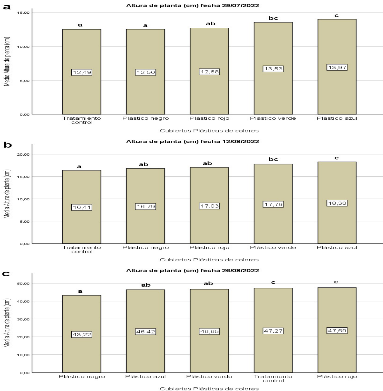
Figura 4. Promedio de altura de planta en los diferentes días después de trasplante: a 10 ddt, b 25 ddt y c 40 ddt
