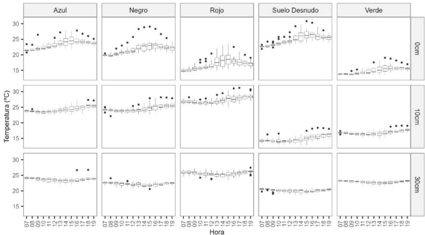
Figura 1. Comportamiento de la temperatura de suelo en los cinco tratamientos de estudio en las profundidades de 0, 10 y 30 cm
