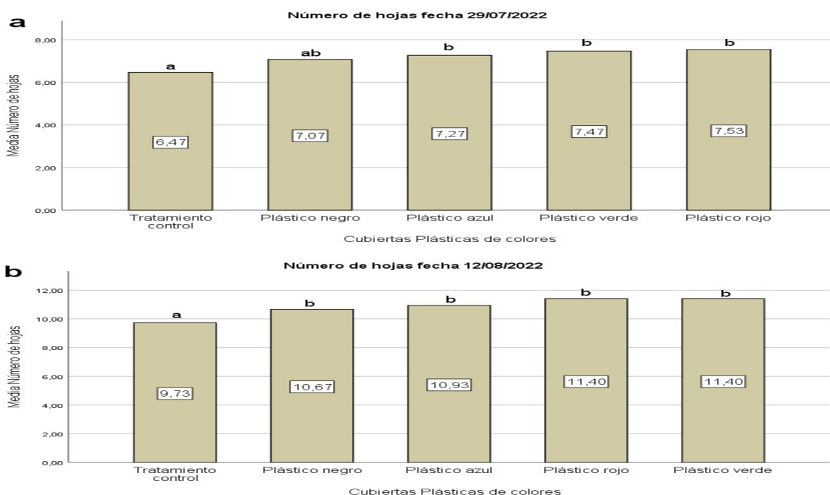
Figura 6. Promedio de número de hojas por planta a diferentes días después de trasplante: a 10 ddt y b 25 ddt
