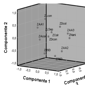
Figura 20: Distribución de los descriptores sobre los tres componentes principales
